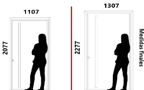
Medidas del Pivot
